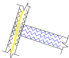
trzystopniowy ściąg na łączeniu panela i liku z zaznaczona trymlinką
